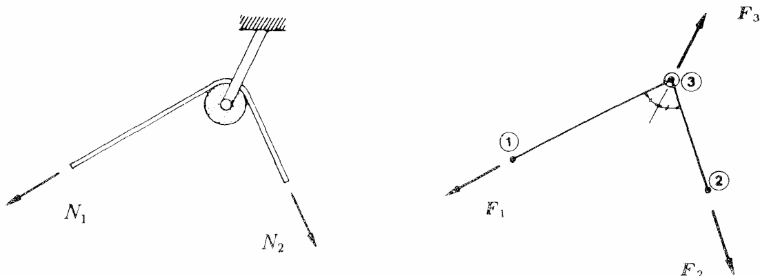
Figura 1. Elemento de cabo ideal (sem atrito)
