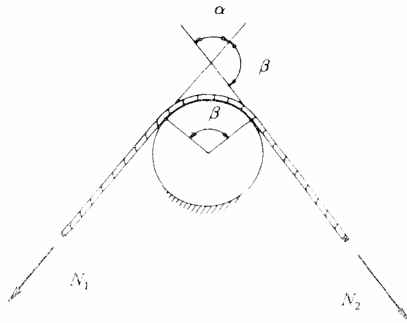
Figura 2. Correia passando por tambor cilíndrico fixo
