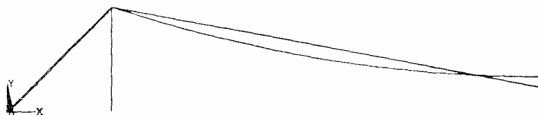
Figura 6. Cabo de ponte pênsil. Geometria inicial (retilínea) e de equilíbrio sob a ação do peso próprio
