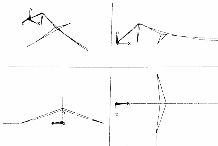
Figura 10. Geometria deformada considerando o escorregamento dos cabos
