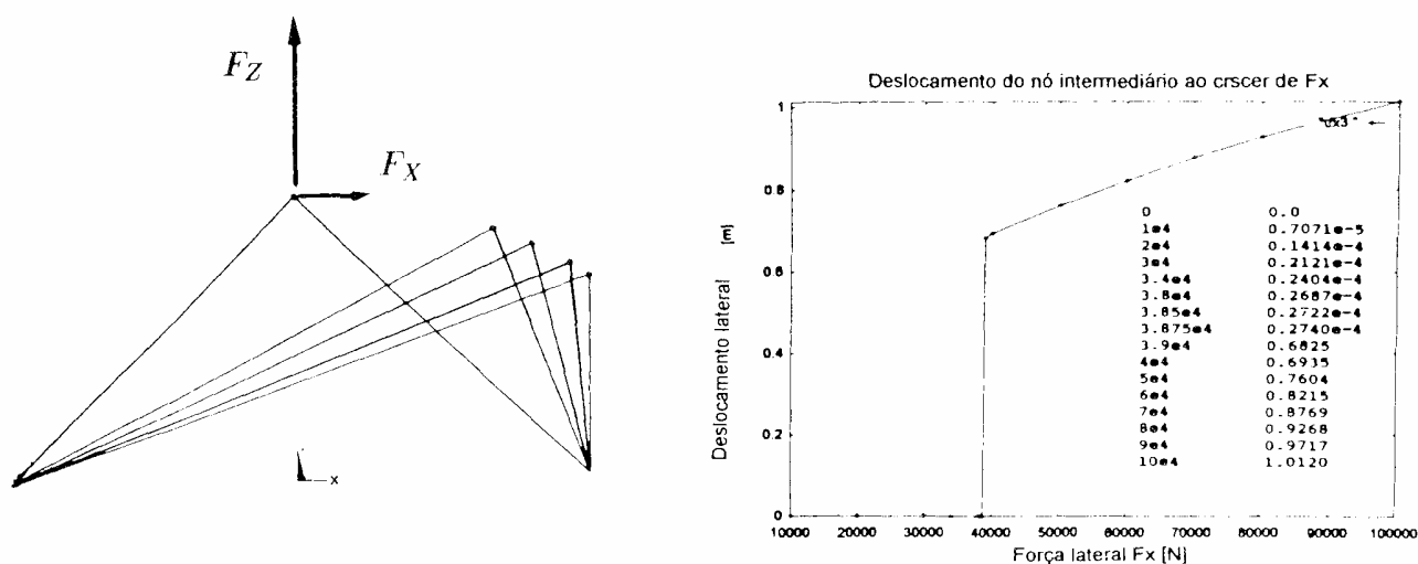
Figura 4. (a) Elemento de cabo escorregando em sucessivas configurações de equilíbrio; (b) Deslocamento do nó intermediário ao crescer de Fx
