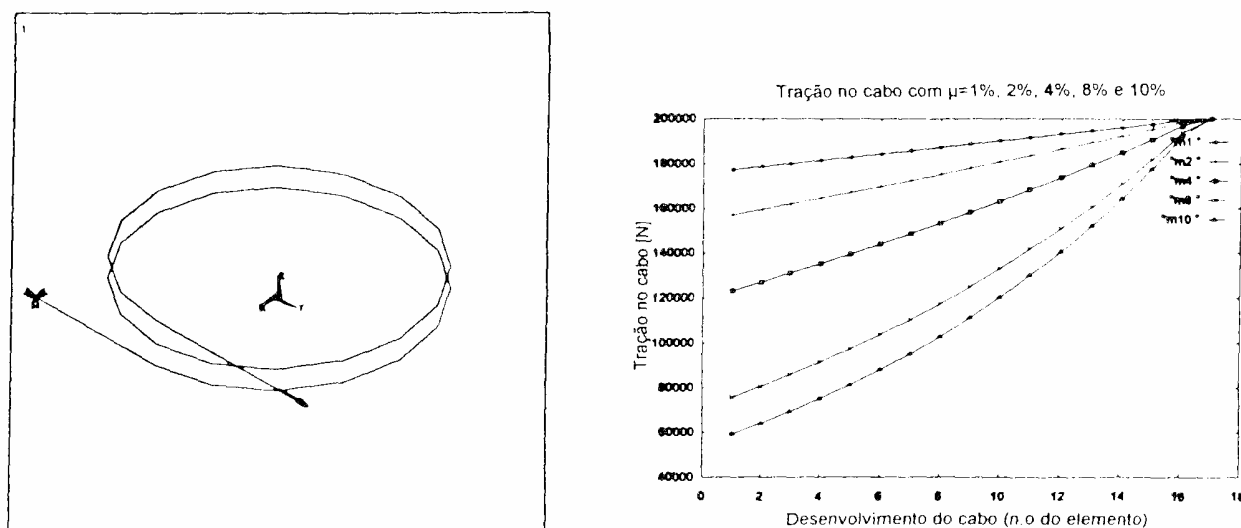
Figura 5. (a) Cabo enrolado a um pilar cilíndrico; (b) Tração no cabo para diversos coeficientes de atrito
