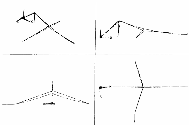
Figura 11. Geometria deformada impedindo o escorregamento dos cabos
